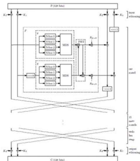
Gambar 1. Struktur Algoritma Twofish
