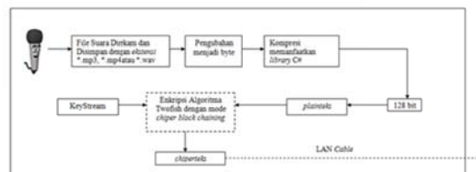
Gambar 3. Proses Enkripsi File Suara
