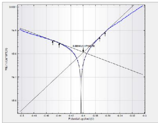
Gambar 1. Grafik Tafel
