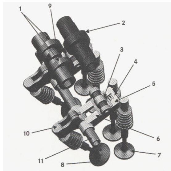
Gambar 6. Mekanisasi pengaturan pembukaan katup [3]
