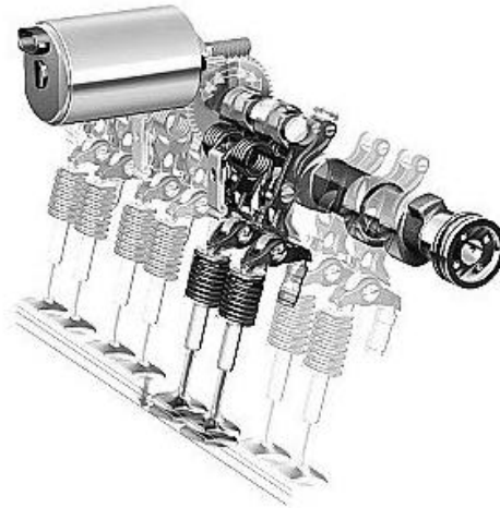
Gambar 9. Mekanisasi Pengatur Katup
