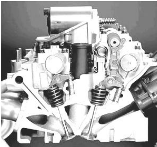
Gambar 11. Mekanisme Valvetronic Terpasang pada Silinder Blok [10]
