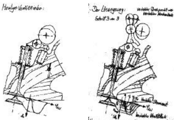
Gambar 8. Pengaturan Katup pada Motor Bakar Bensin
