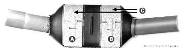
Gambar 5. Penampung Katalisator 3 Jalan
