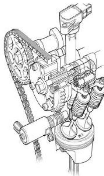
Gambar 7. Sistem Pengaturan Katup Menurut Desain VTEC
