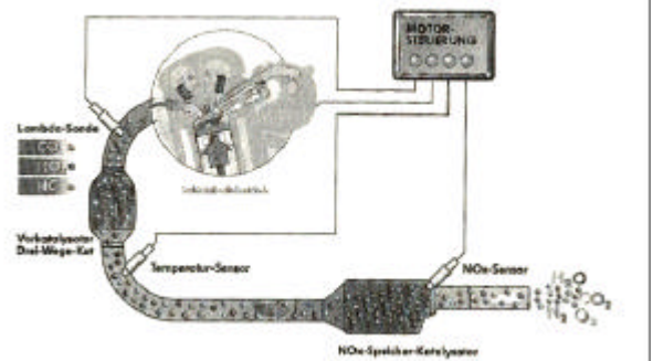
Gambar 3. Skema Pengolahan Gas Buang pada Campuran yang Kurus [2]
