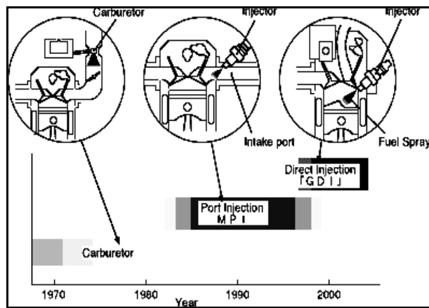
Gambar 1. Skema Tiga Jenis Penyemprotan Bahan Bakar
