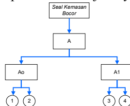
Gambar 4 Diagram Pohon Kesalahan Bentuk Seal Kemasan Bocor
