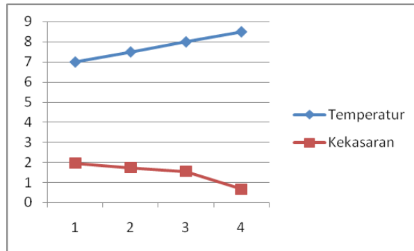
Gambar 6. Grafik kekasaran pengecoran II (Sumber: data diolah)
