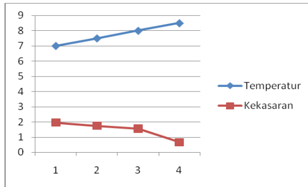
Gambar 7. Grafik kekasaran pengecoran III (Sumber: data diolah)
