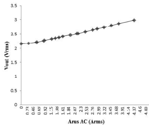
Gambar 10. Karakteristik tegangan keluaran (Vout) sensor arus terhadap perubahan arus yang diukur.
