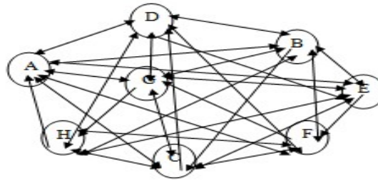
Gambar 3. Graf Lintasan Distribusi Awal Perusahaan (Sumber: Data Perusahaan)
