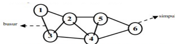
Gambar 1 Graph dengan 6 verteks dan 7 edge.
