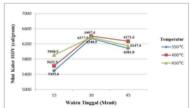
Gambar 8. Grafik Hasil Nilai Kalor Biobriket Komposisi 75% Kulit Mete – 25% Sekam Padi.
