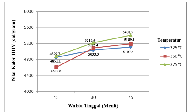
Gambar 7. Grafik Hasil Nilai Kalor Biobriket Komposisi 50% Kulit Mete – 50% Sekam Padi.
