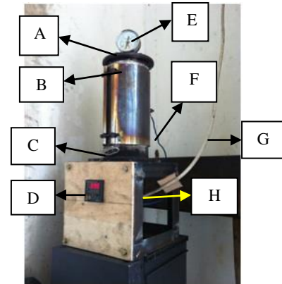
Gambar 6. Instalasi Alat - Alat Uji Pirolisa.
