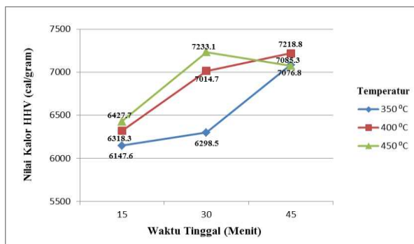
Gambar 9. Grafik Hasil Nilai Kalor Biobriket Komposisi 100% Kulit Mete.
