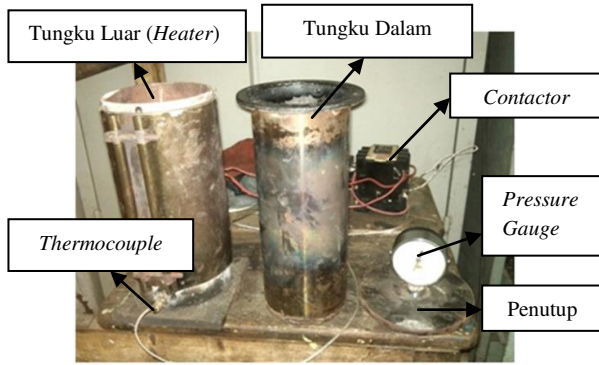
Gambar 2. Tungku Pirolisa
