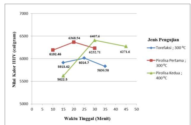
Gambar 12. Grafik Analisa Perbandingan Hasil Nilai Kalor Pada 3 Macam Pengujian Biobriket Campuran 75% Kulit Mete – 25% Sekam Padi.
