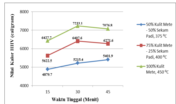
Gambar 10. Grafik Hasil Nilai Kalor Terbaik Biobriket Dari 3 Variasi Komposisi, Temperatur, Dan Waktu Tinggal.
