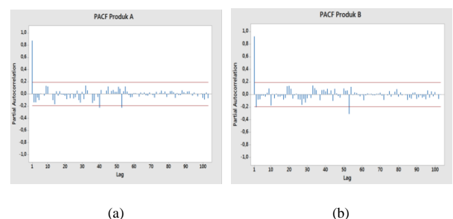
Gambar 3. Uji PACF produk A dan produk B
