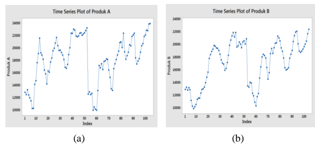
Gambar 1. Plot data penjualan produk A dan produk B
