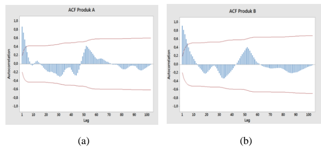
Gambar 2. Uji ACF produk A dan produk B
