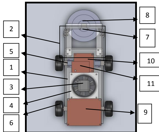
Gambar 4. Desain Prototype Robot Pembersih Kaca
