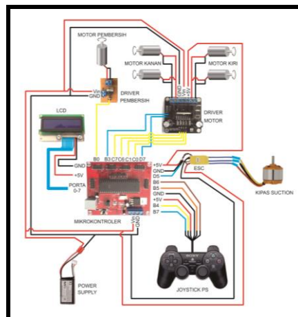
Gambar 5. Desain hardware Elektronik Prototype Robot Pembersih Kaca
