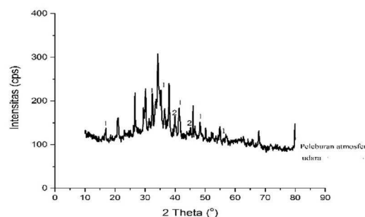
Gambar 1. Difraktogram padatan abu dasar hasil leburan (1=Natrium Silikat, 2= Natrium AluminatSilikat)
