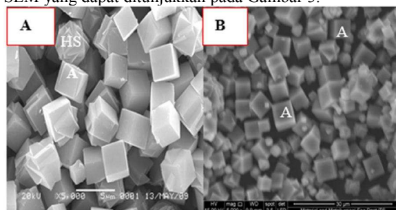
Gambar 3. Hasil Foto SEM (a) Zeolit-A tanpa pemisahan Fe dan Ca [3] (b) Zeolit-A dengan pemisahan Fe dan Ca (A=Zeolit-A, HS=Hidroksi Sodalit)
