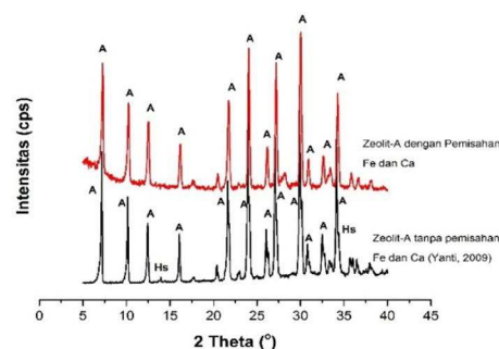
Gambar 2. Difraktogram Zeolit-A tanpa pemisahan Fe dan Ca [3] dan Zeolit-A hasil sintesis dengan pemisahan Fe dan Ca
