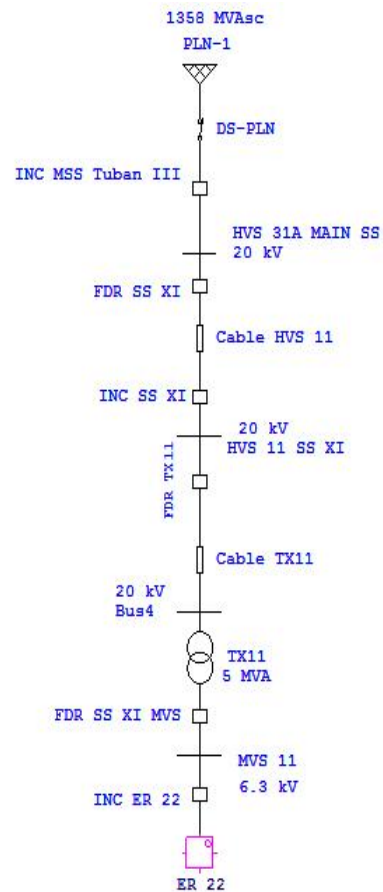
Gambar 1 Single Line Diagram penyulang 1 pabrik semen Tuban beserta pembagian saluran dan load point
