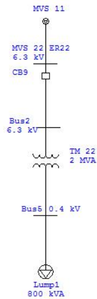
Gambar 3 Single Line Diagram load point ER 22 penyulang 1 pabrik semen Tuban
