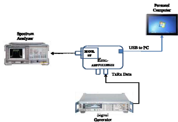
Gambar 6. Skema Pengukuran dengan Input Sinyal Generator
