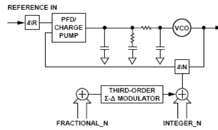
Gambar 2. Rangkaian PLL ADF7021-N
