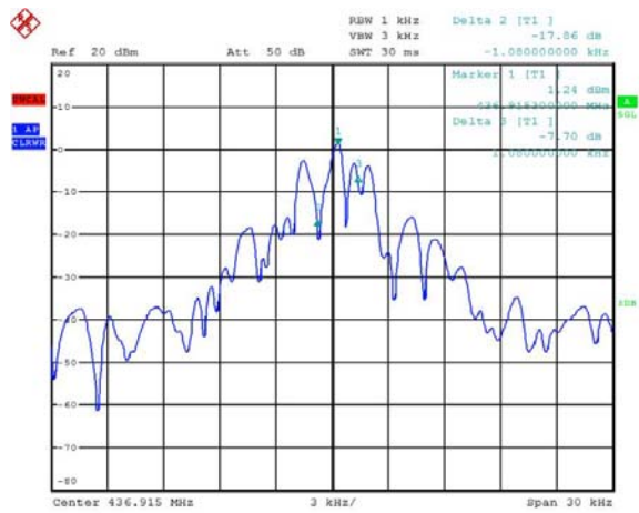
Gambar 10. Spektrum Sinyal FSK dengan Input Sinyal PN9
