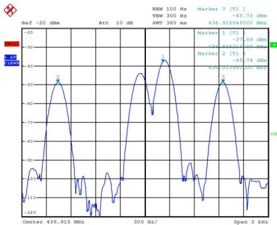
Gambar 7. Spektrum FSK dengan Input Daya 13dBm
