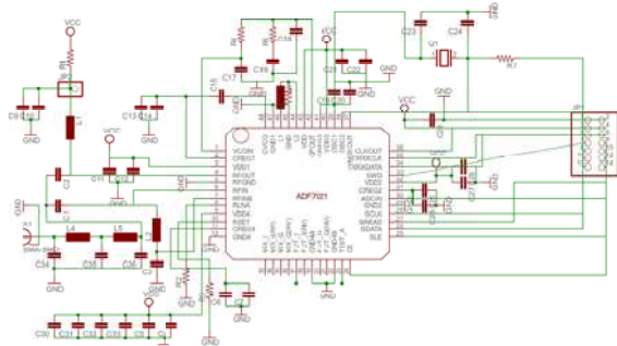
Gambar 4. Skematik Modulator FSK 9600 Baud
