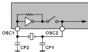
Gambar 1. Rangkaian Osilator pada ADF7021-N
