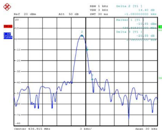
Gambar 9. Sinyal Space dari Tone -ve
