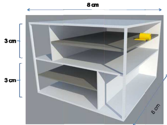
Gambar 6. Sketsa 3D Payload Komunikasi Satelit IiNUSAT-01
