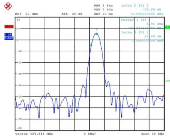
Gambar 8. Sinyal Mark dari Tone +ve
