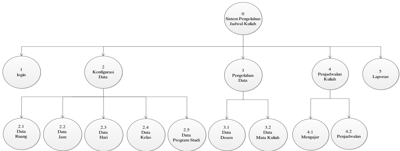
Gambar 3. Diagram Berjenjang
