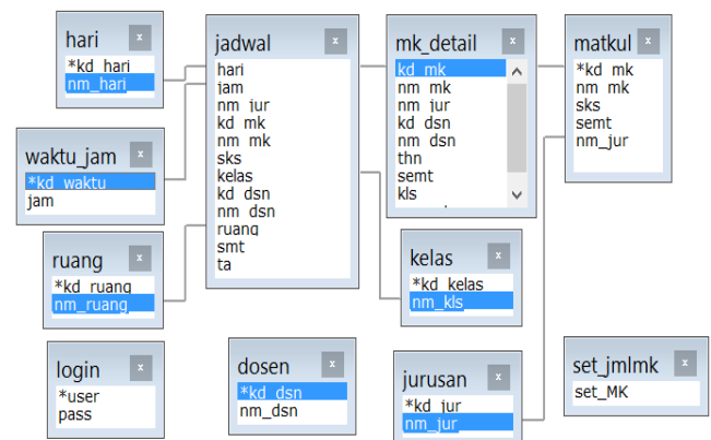
Gambar 6. Perancangan Relasi Tabel
