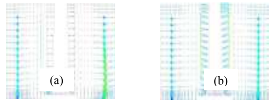
Gambar 4. Pola sirkulasi aliran fluida masuk (a) membran sebagai black box , dan (b) membran sebagai porous media
