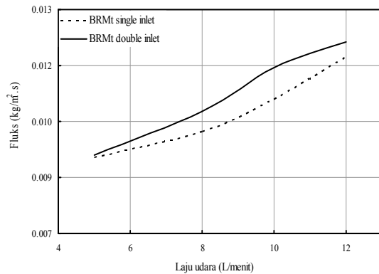
Gambar 12. Hubungan fluks dengan perubahan laju udara pada BRMt, membran sebagai porous media
