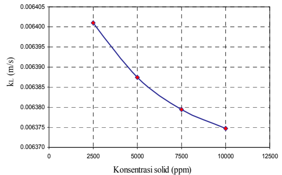
Gambar 11. Hubungan laju transfer massa gas-liquid ( k_L ) dengan perubahan konsentrasi solid dengan membran sebagai black box
