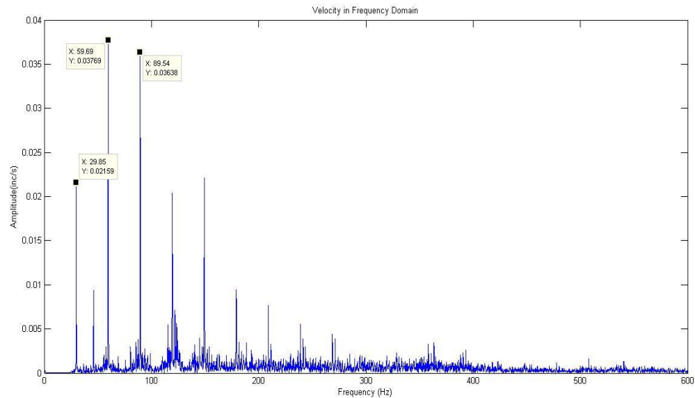
Gambar 12. Sinyal FFT kopling roda gigi kondisi misalignment arah radial horisontal dalam domain frekuensi pada 1800 rpm.
