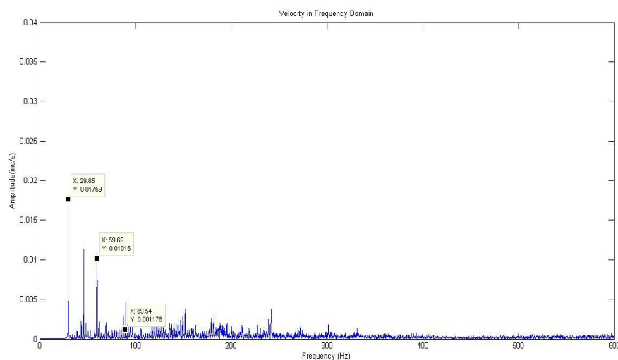
Gambar 16. Sinyal FFT kopling beam kondisi alignment arah radial horizontal dalam domain frekuensi pada 1800 rpm.
