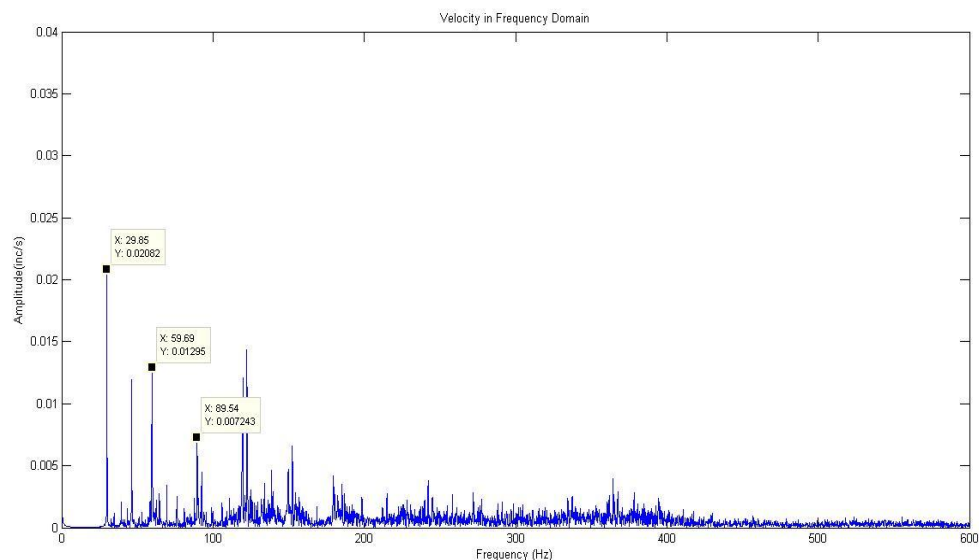
Gambar 13. Sinyal FFT kopling roda gigi kondisi alignment arah radial horisontal dalam domain frekuensi pada 1800 rpm.
