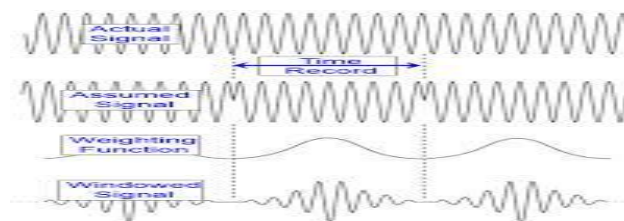
Gambar 6. Efek window pada time domain
