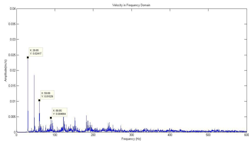
Gambar 15. Sinyal FFT kopling beam kondisi misalignment arah radial horizontal dalam domain frekuensi pada 1800 rpm.
