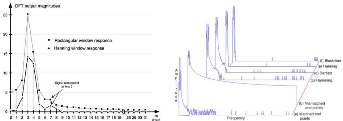
Gambar 7. Perbandingan hanning window dengan jenis window lainnya
