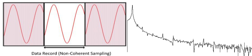
Gambar 5. Kebocoran ( Leak ) terjadi pada gelombang sinusoidal
