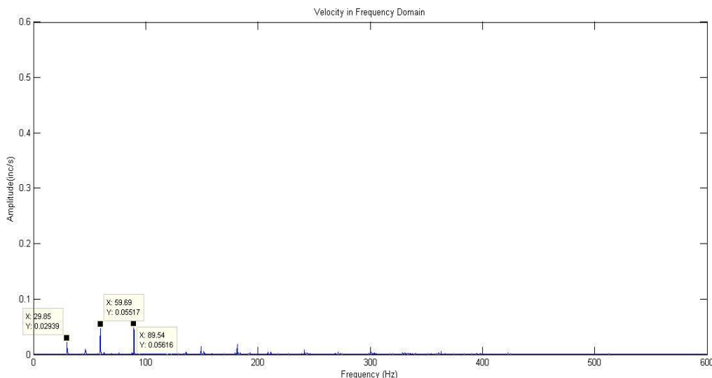
Gambar 10. Sinyal FFT kopling jaw kondisi alignment arah radial horisontal dalam domain frekuensi pada 1800 rpm.
