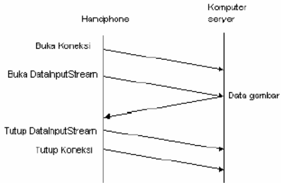
Gambar 6. Time Sequence Diagram Koneksi Jaringan untuk Download
