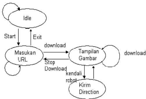
Gambar 5. State Diagram Interaksi User dengan Handphone
