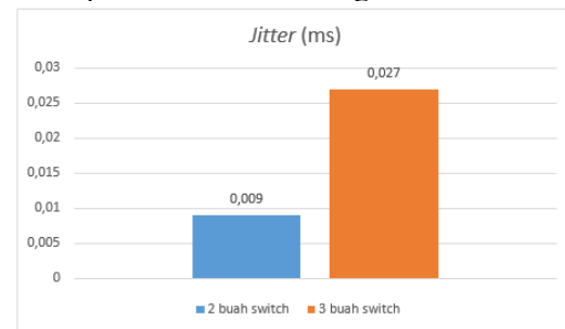
Gambar 8. Grafik Jitter
