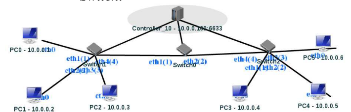
Gambar 2. Skenario 2 Menggunakan 3 Buah Switch
