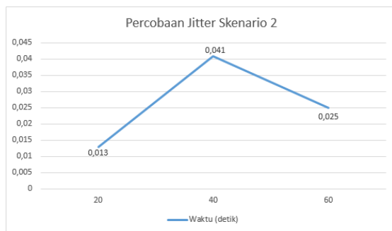
Gambar 6. Grafik Jitter Skenario 2
