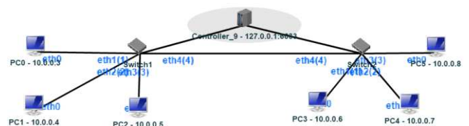
Gambar 1. Skenario 1 Menggunakan 2 Buah Switch
