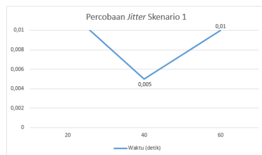
Gambar 4. Grafik Jitter Skenario 1
