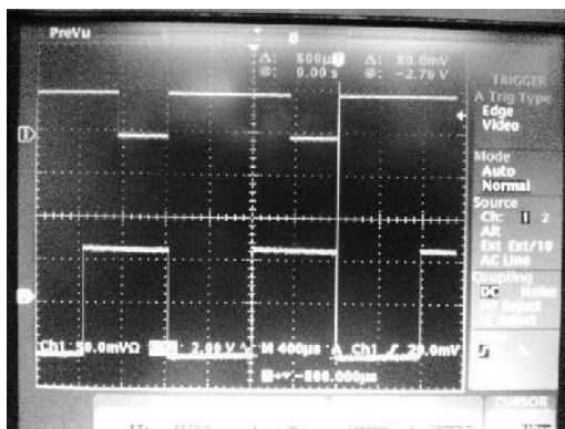
Gambar9. Hasil pengujian modulator-demodulator (CCITT V.23) (1: sinyal digital yang diterima; 2: sinyal digital yang dikirim)
