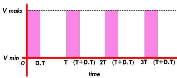
Gambar 3. Bentuk gelombang pulsa PWM
