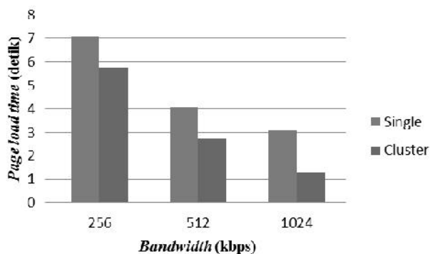
Gambar. 2. Perbandingan page load time antara server LMS single dengan server LMS cluster.
