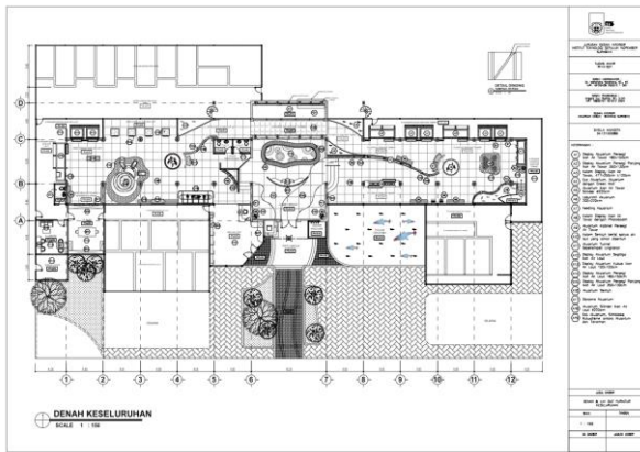
Gambar 2. Layout keseluruhan akuarium KBS
