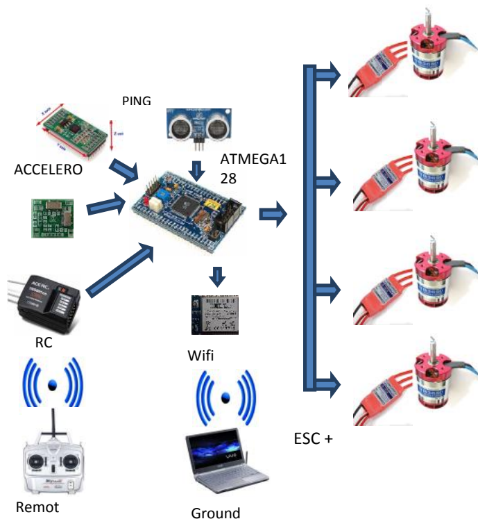
Gambar 5 Rancangan Sistem Elektronika Quadcopter
