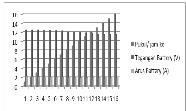
Gambar 6. Plotting Arus Terhadap Lama Waktu Pembebanan Lampu
