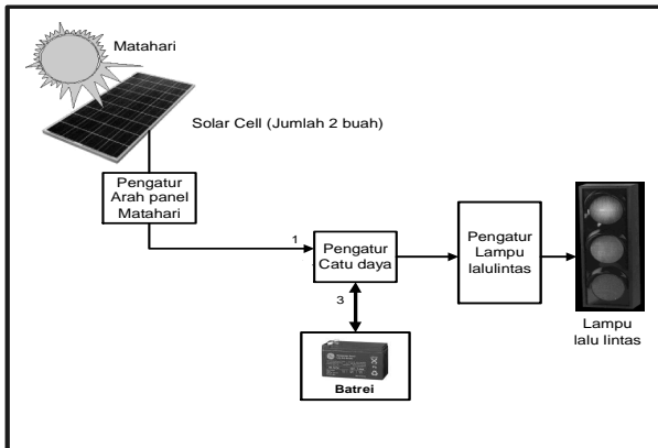
Gambar 3. Rancangan Sistem Lampu Lalu lintas dengan Tenaga Energi Matahari
