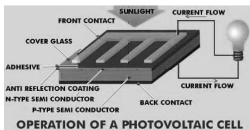
Gambar 1. Konstruksi Dasar Fotovoltaik
