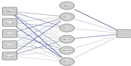
Gambar 2. Arsitektur NN 5 Neuron Data Produksi Minyak Bumi
