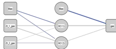
Gambar 4. Arsitektur NN 2 Neuron Data Produksi Gas Bumi
