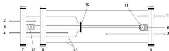
Gambar 1. Skema pengujian elektrokimia untuk pengukuran konduktivitas ion sel elektrolit.
