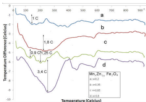
Gambar 6. Hasil pengujian karakteristik termal \text{Mn}_x\text{Zn}_{1-x}\text{Fe}_2\text{O}_4 dengan menggunakan DTA.
