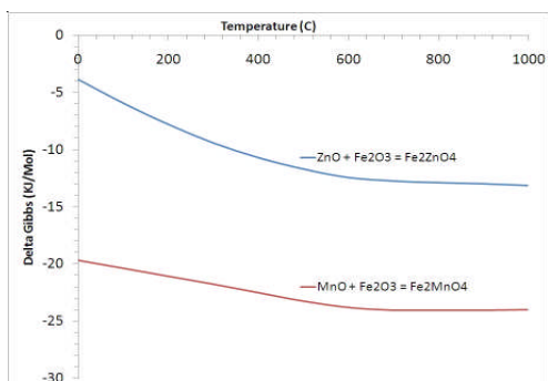
Gambar 5. Kurva simulasi \Delta G (energi bebas Gibbs ) reaksi pembentukan \text{Fe}_2\text{MnO}_4 dan \text{Fe}_2\text{ZnO}_4 .
