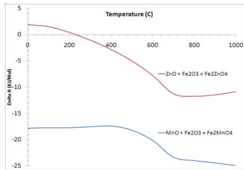
Gambar 4. Kurva simulasi \Delta H (entalpi) reaksi pembentukan \text{Fe}_2\text{MnO}_4 dan \text{Fe}_2\text{ZnO}_4 .
