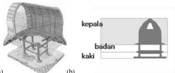
Gambar 7. Lumbung Padi Sasak (a). Penampang (b). Hirarki
