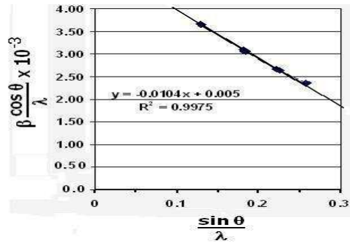
Gambar 4. Grafik hubungan linier antara \beta \cdot \cos\theta/\lambda terhadap \sin\theta/\lambda pada \text{LaMnO}_{3,0} .
