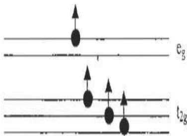
Gambar 3. Konfigurasi elektron \text{Mn}_{4+} dalam medan elektronik kristal oktahedral.
