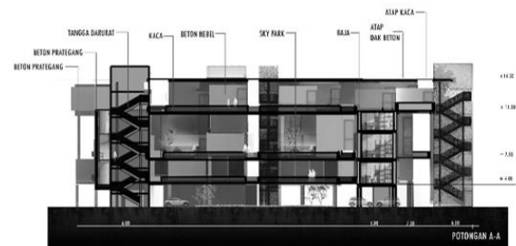
Gambar 6. Potongan bangunan
