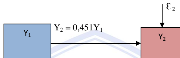
Gambar 4. Hubungan Empiris Sub Struktur 2 ( Y_1 terhadap Y_2 )
