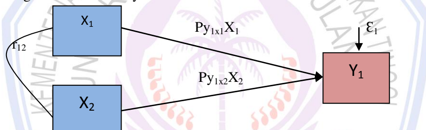
Gambar 1. Hubungan Sub Struktur 1 ( X_1 dan X_2 terhadap Y_1 )
