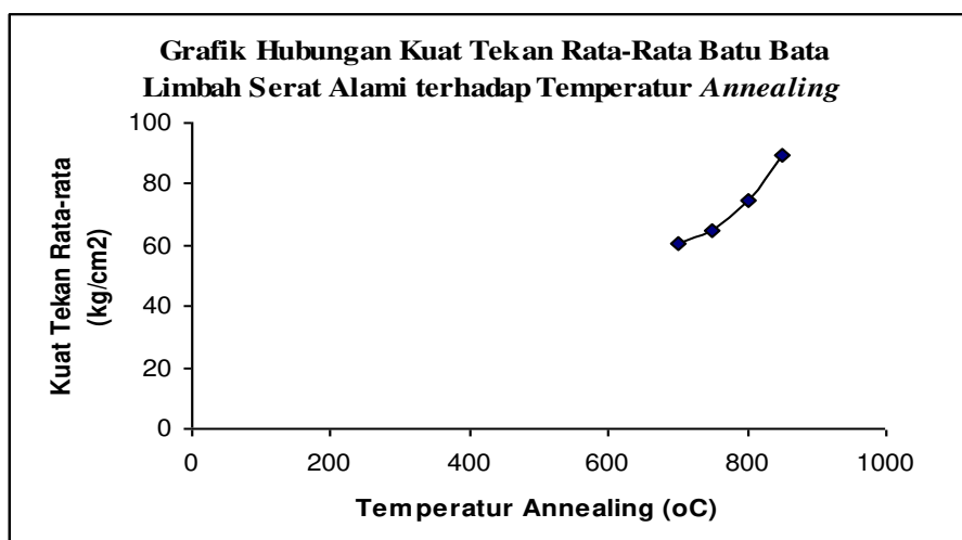
Gambar 1. Grafik hubungan kuat tekan rata-rata batubata limbah serat alami terhadap variasi temperatur Annealing .
