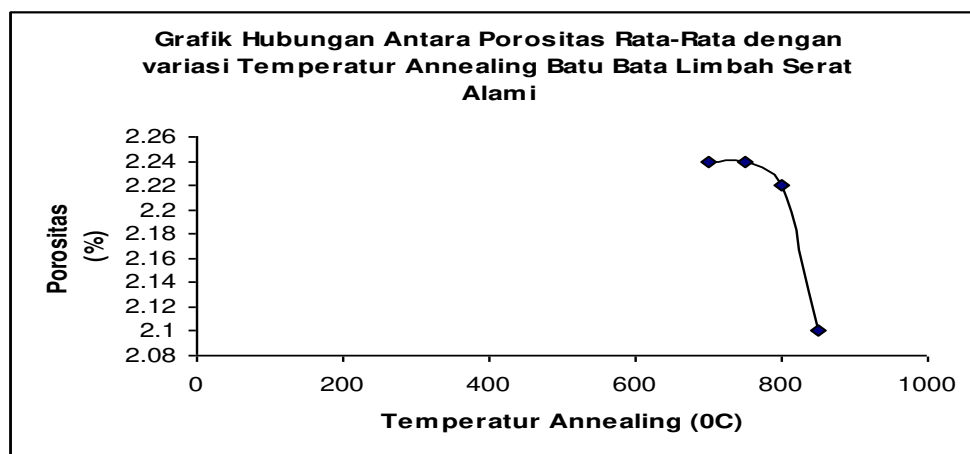
Gambar 12. Grafik hubungan porositas rata-rata dengan temperatur Annealing batu bata limbah serat alami
