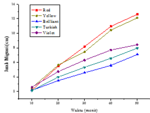
Gambar 5. Pengaruh waktu elektroforesis terhadap jarak migrasi remazol
