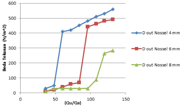
Gambar 7. Grafik hubungan Q_u/Q_a terhadap beda tekanan pada debit air 5 liter/menit.
