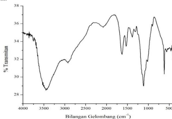
Gambar 3.3 Spektrogram FTIR Membran Komposit Kitosan/ Monmorillonit Termodifikasi Silan 10%
