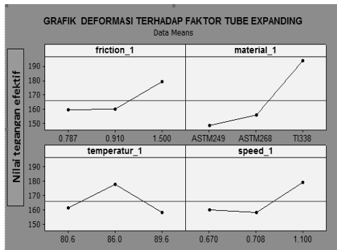
Gambar 7. Grafik deformasi terhadap faktor tube expanding .
