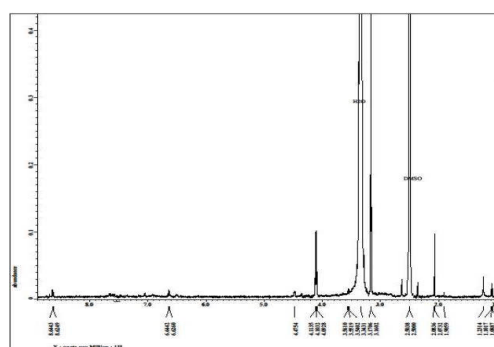
Gambar 3. Hasil pemeriksaan 1 H-NMR terhadap EDA-folat
