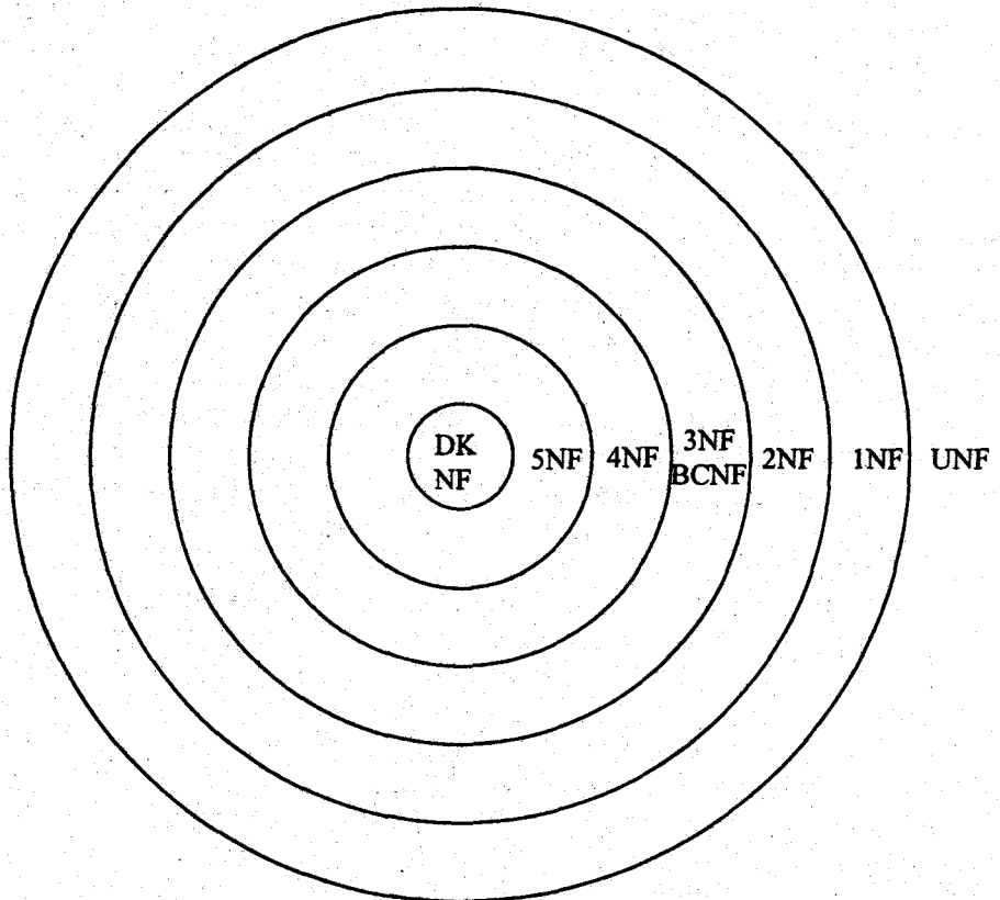
Gambar 1. Tingkat-tingkat Bentuk Normal
