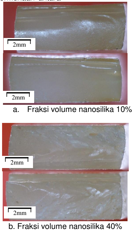
Gambar 5. Foto makro penampang patah komposit nanosilika-phenolic
