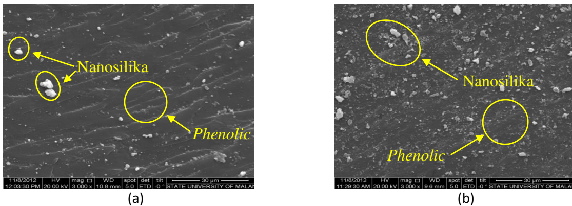
Gambar 6. SEM pengujian impak dengan fraksi volume nanosilika (a) 10%, (b) 40%
