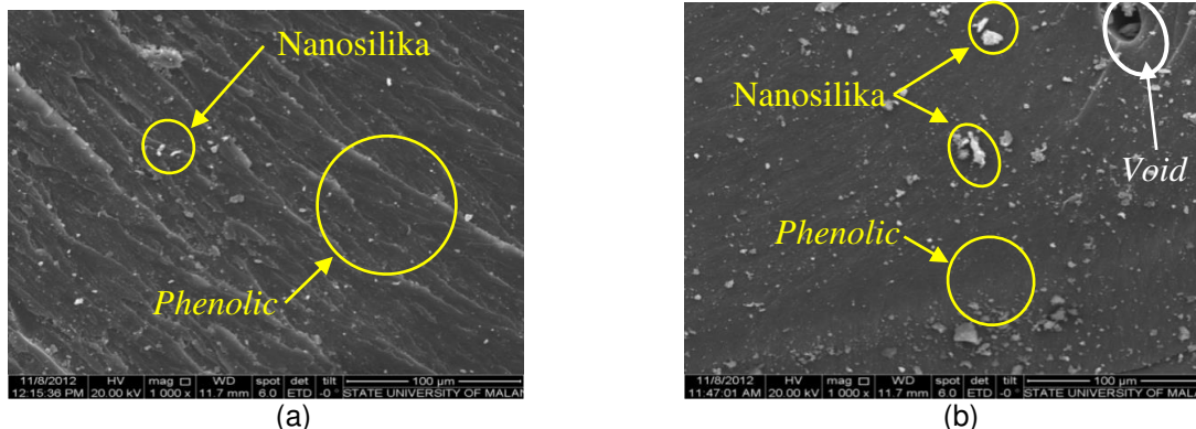
Gambar 3. SEM penguji bending dengan fraksi volume nanosilika (a) 30% (b) 60%
