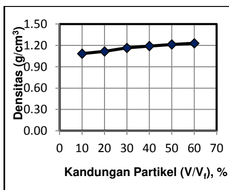
Gambar 7. Grafik densitas komposit
