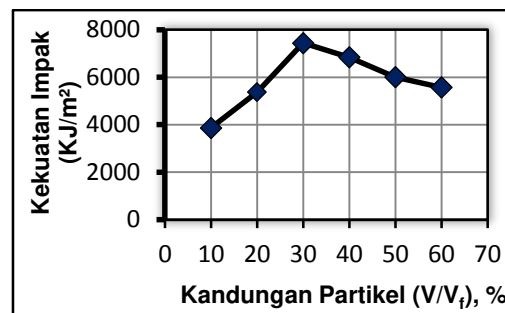
Gambar 4. Grafik ketangguhan impak
