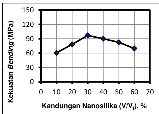
Gambar 1. Kekuatan bending
