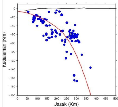
Gambar 11. Cross Section sesudah relokasi
