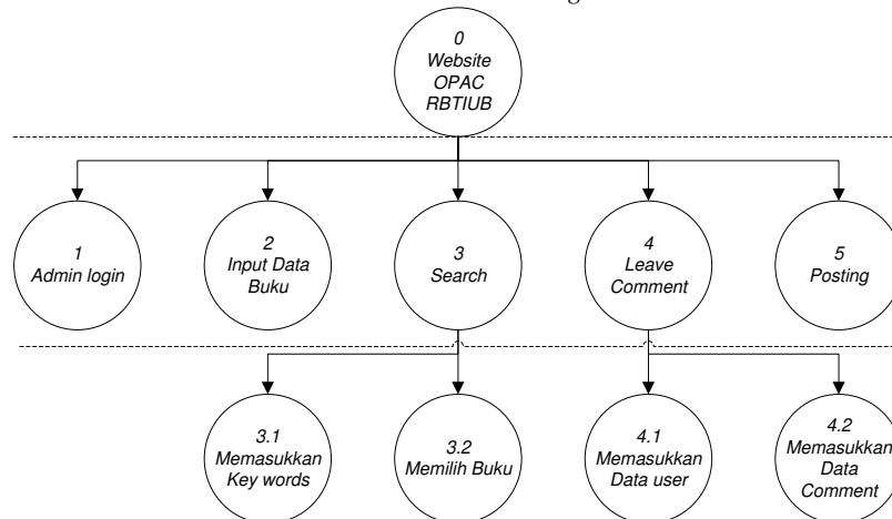
Gambar 2 Bagan Berjenjang DFD
