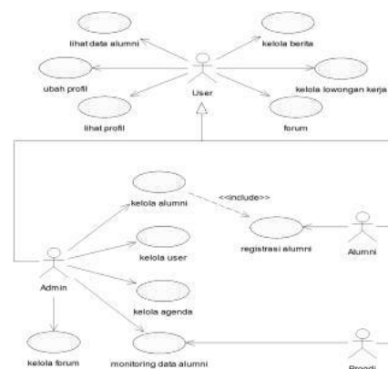
Gambar 1 : Use Case Diagram Sistem Pelacakan
