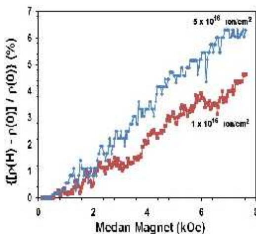
Gambar 4. Kurva Magnetoresistance lapisan tipis C/Si hasil implan ion Ni^+ dan Ar^+
