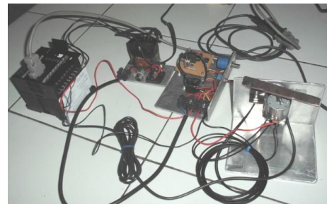
Gambar 4 Rangkaian keseluruhan pengukur kecepatan motor DC berbasis PLC
