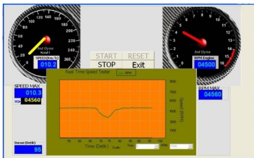
Gambar 9 Pengujian kecepatan 1
