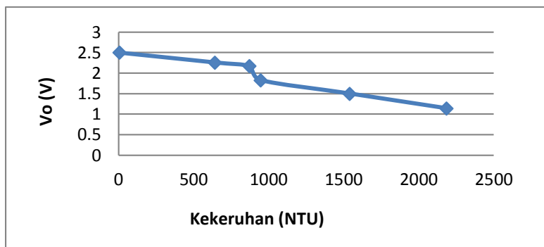
Gambar 12. Hubungan tegangan keluaran sensor LDR dengan kekeruhan
