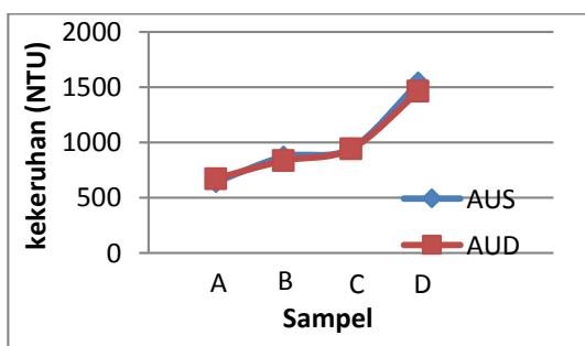
Gambar 14. Plot pengukuran kekeruhan menggunakan AUD dan AUS
