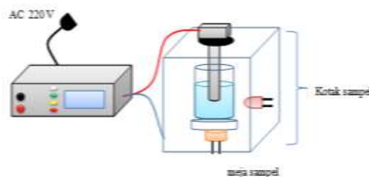
Gambar 4. Desain mekanik sistem alat ukur salinitas dan kekeruhan
