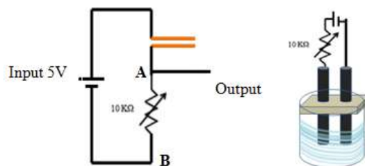
Gambar 1. Ilustrasi rangkaian sensor salinitas
