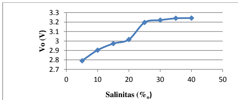
Gambar 11. Hubungan tegangan keluaran sensor elektroda dengan salinitas
