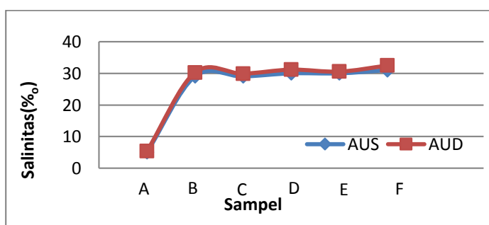
Gambar 13. Plot pengukuran salinitas menggunakan AUD dan AUS
