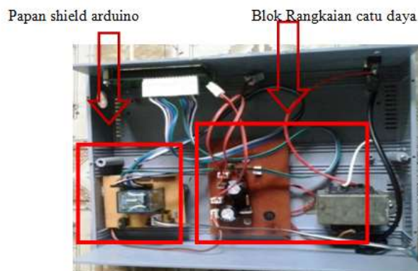
Gambar 9. Foto hasil desain rangkaian elektronika sistem alat ukur
