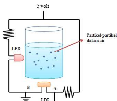
Gambar 2. Rangkaian aplikasi sensor kekeruhan
