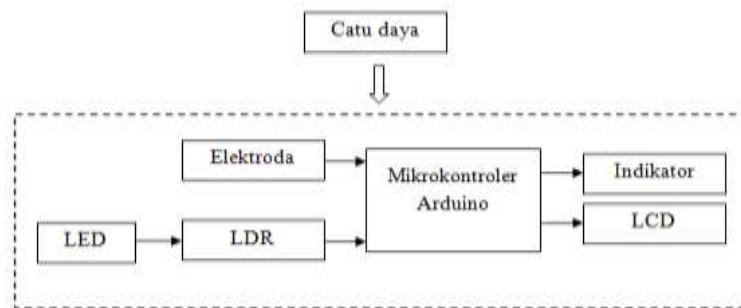
Gambar 3. Blok diagram alat ukur salinitas dan kekeruhan.
