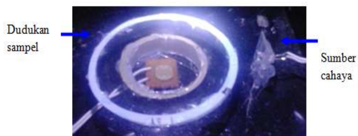
Gambar 7. Foto posisi sensor kekeruhan pada dasar kotak sampel
