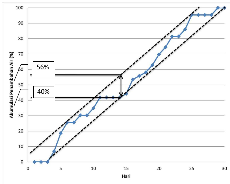
Gambar 2. Persentase Penambahan Air pada Kadar Air Pengomposan 60%
