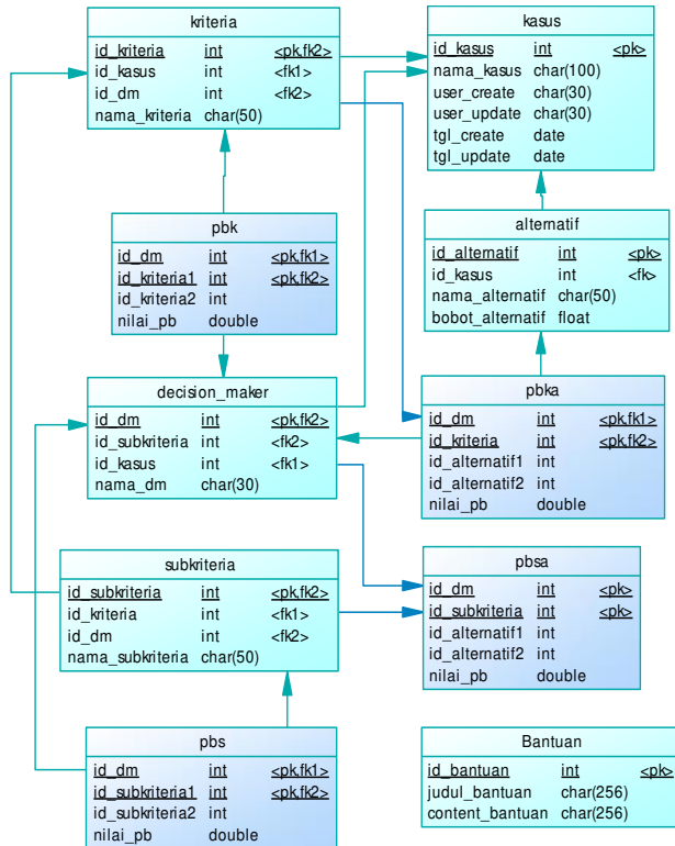
Gambar 4. Database Arsitektur
