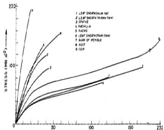
Gambar 4. Kekuatan tarik beberapa bagian kelapa termasuk serat sabut kelapa,[11].
