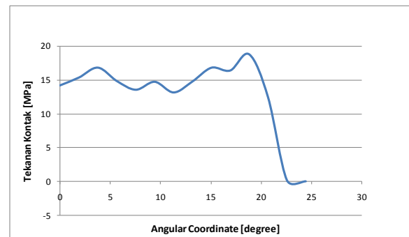
Gambar 3. Distribusi tekanan kontak CoCr-on-CoCr
