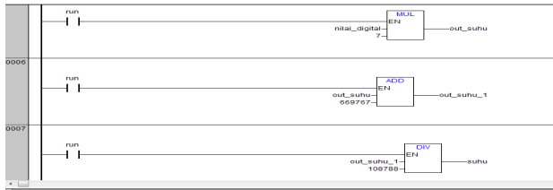
Gambar 17. Tampilan pemrograman ladder diagram untuk pembacaan suhu
