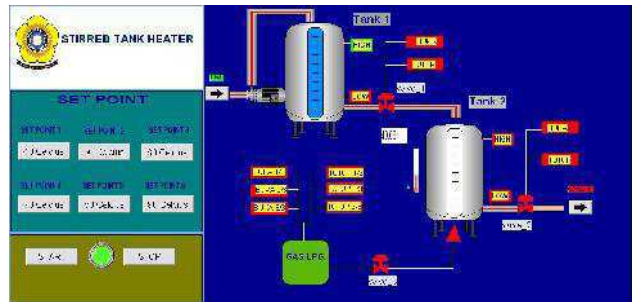
Gambar 16. Tampilan sistem SCADA setelah proses selesai
